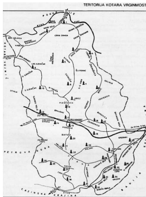
Срез Вргинност 60
